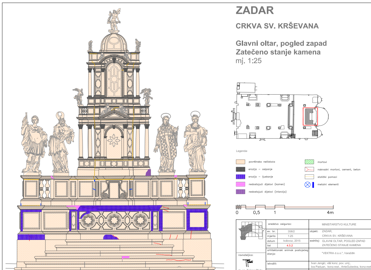
Zadar, crkva sv. Krševana. Arhitektonska snimka postojećeg stanja zapadne strane glavnog oltara s mapiranim oštećenjima. Izrada: Vektra d.o.o., B. Milković, 2019.
