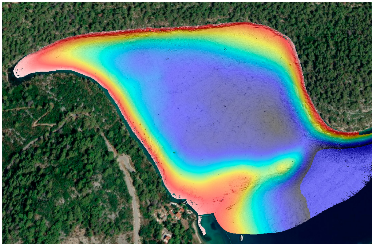
Dubrovačko-neretvanska županija, podmorje, rezultati batimetrijskog mjerenja uvale Polače. Izrada: Helicop, 2025.
