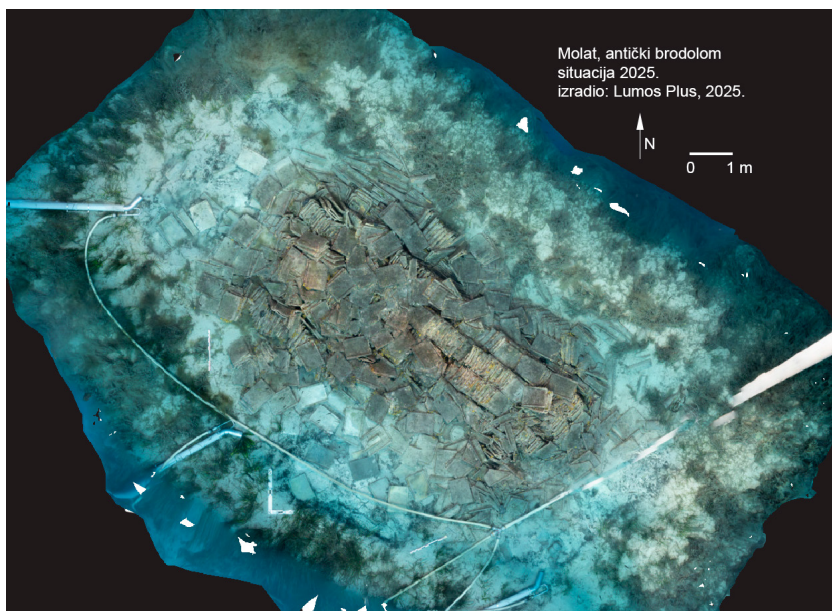
Otok Molat, antički brodolom, ortofotografija nalazišta. Izrada: Lumos plus, 2025.
