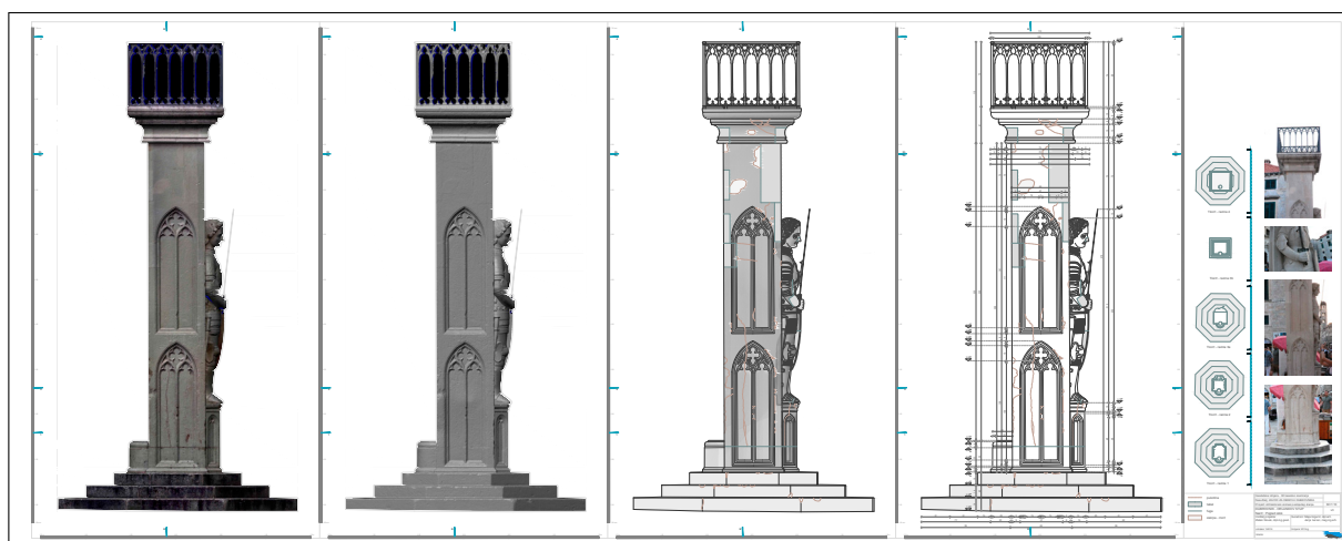
Dubrovnik, Orlandov stup. Arhitektonska snimka postojećega stanja, pogled s istoka. Izrada: Vektra d.o.o., 2014.
