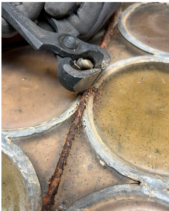
Poreč, Eufrazijeva bazilika (katedrala Uznesenja Marijina). Radovi demontaže izvornih staklenih okulusa iz olovne mreže. Snimka: R. Mijalić, 2025.
