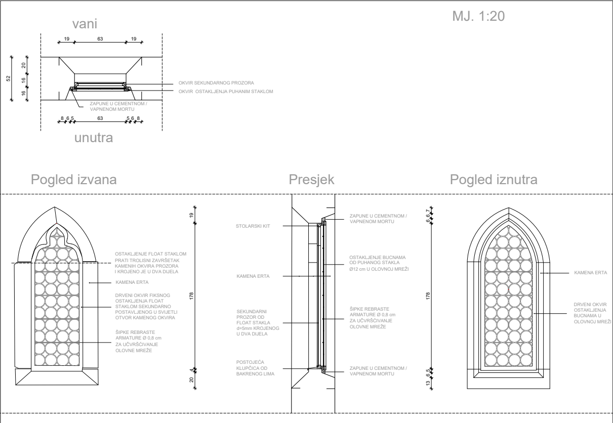
Poreč, Eufrazijeva bazilika (katedrala Uznesenja Marijina). Arhitektonska snimka postojećega stanja južnih prozora glavnog broda. Izrada: B. Milković, 2025.
