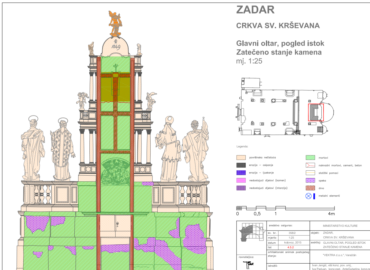
Zadar, crkva sv. Krševana. Arhitektonska snimka postojećeg stanja istočne strane glavnog oltara s mapiranim oštećenjima. Izrada: Vektra d.o.o., B. Milković, 2019.
