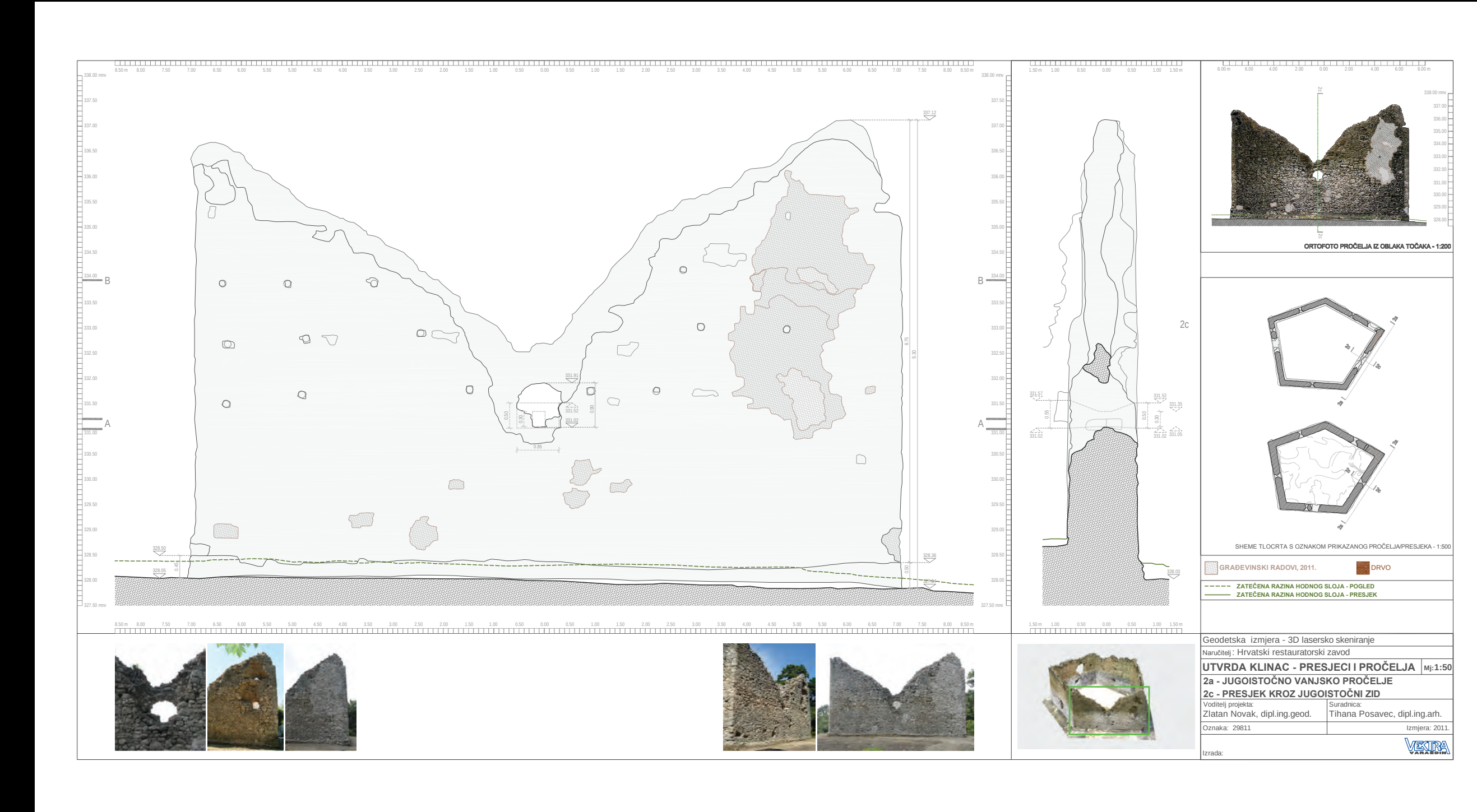
Nacrtna dokumentacija jugoistočnog pročelja utvrde Klinac. Snimak: "Vektra-Geo3D d.o.o.", 2011.
