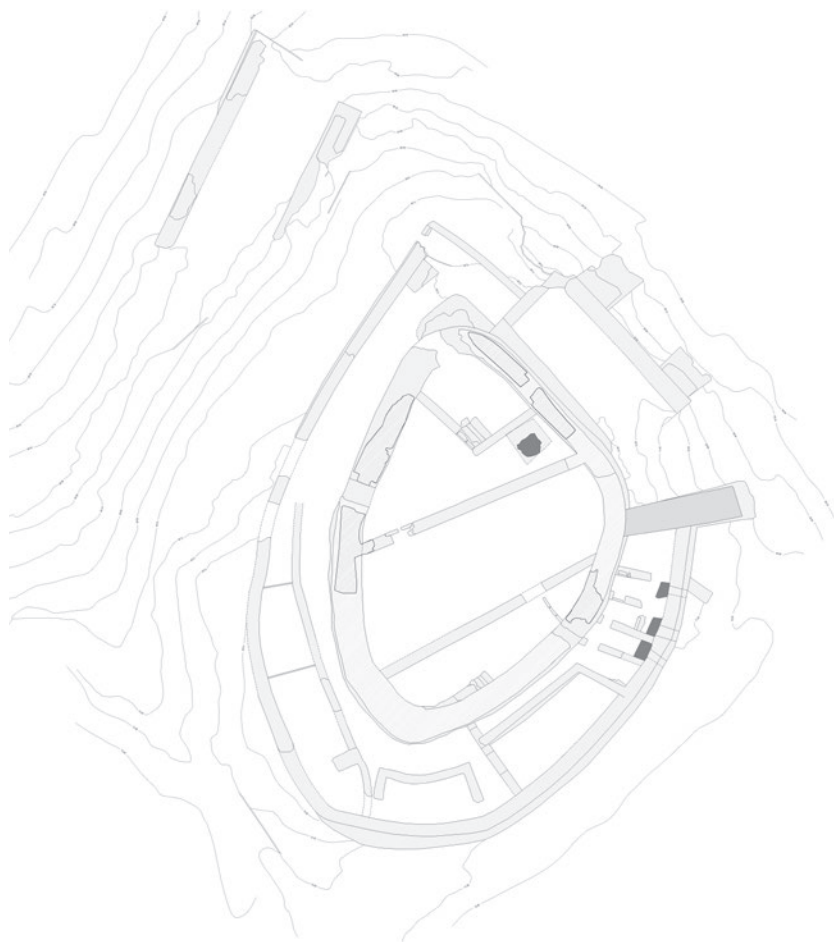
Tlocrt gradine Badanj, Vektra d.o.o., 2013.
