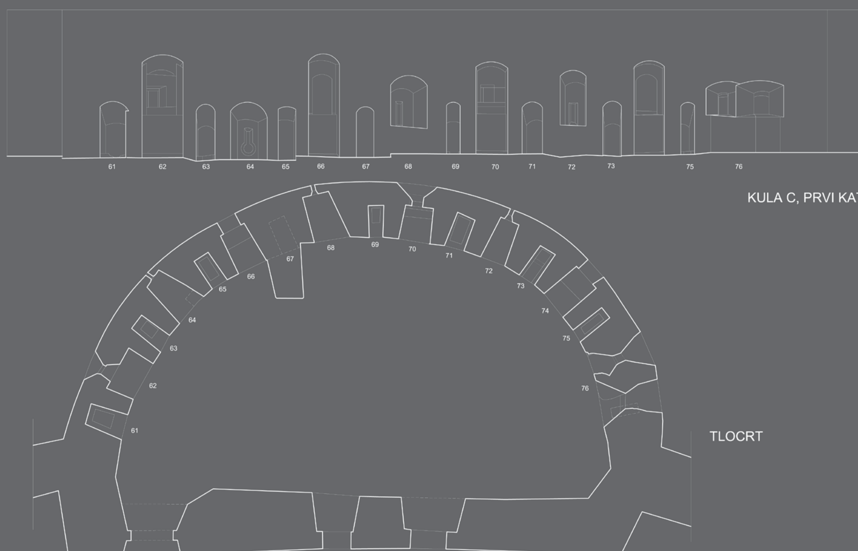
Prvi kat (kapela), pogled na razvijeni plašt i tlocrt pročelnog zida s nišama strijelnica.
