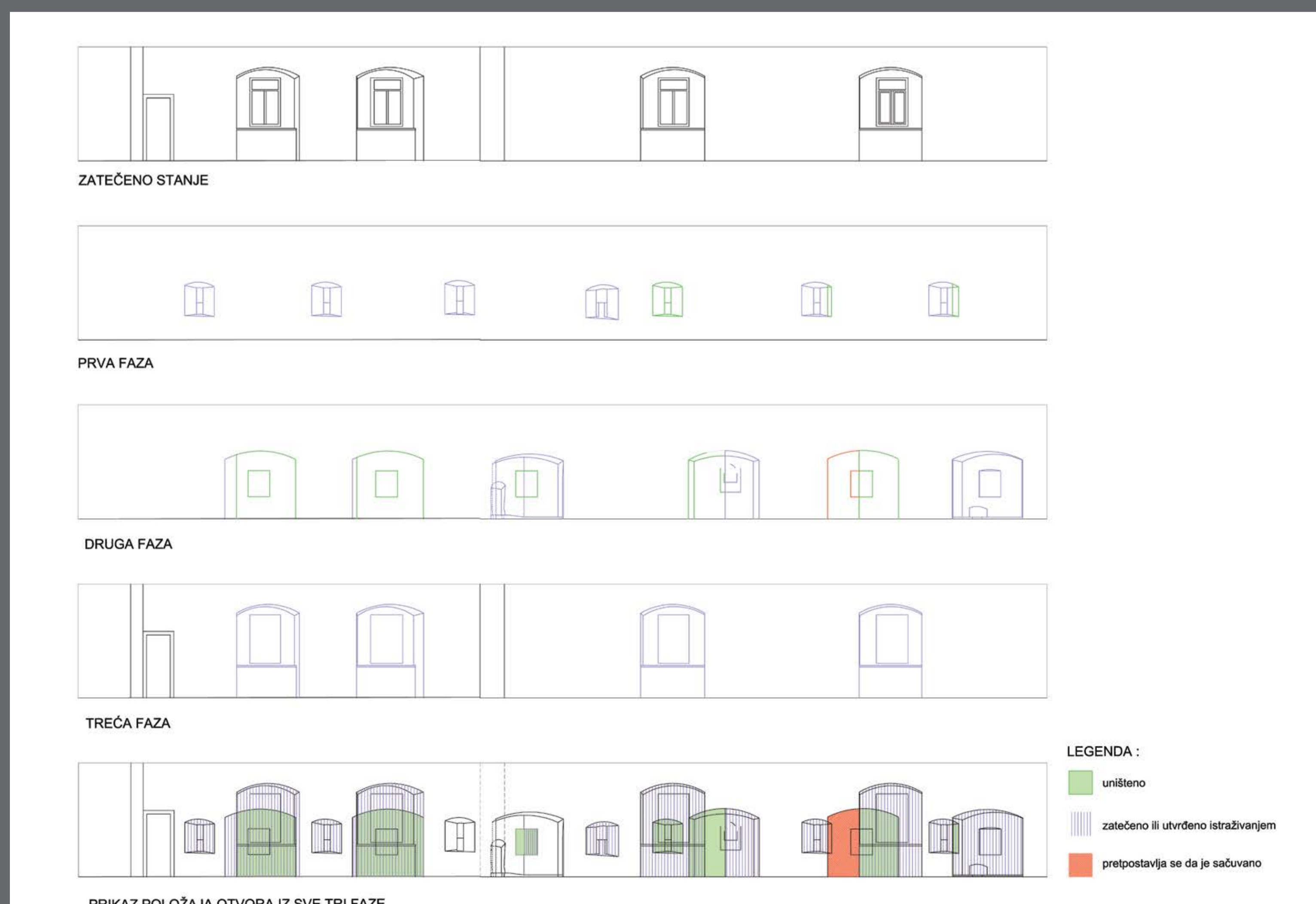
Drugi kat, unutrašnjost, razvijeni plašt obodnog zida kule, razvojne faze.
