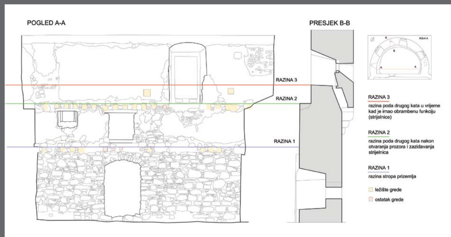
Unutrašnjost kule, razine ranijih etaža.
