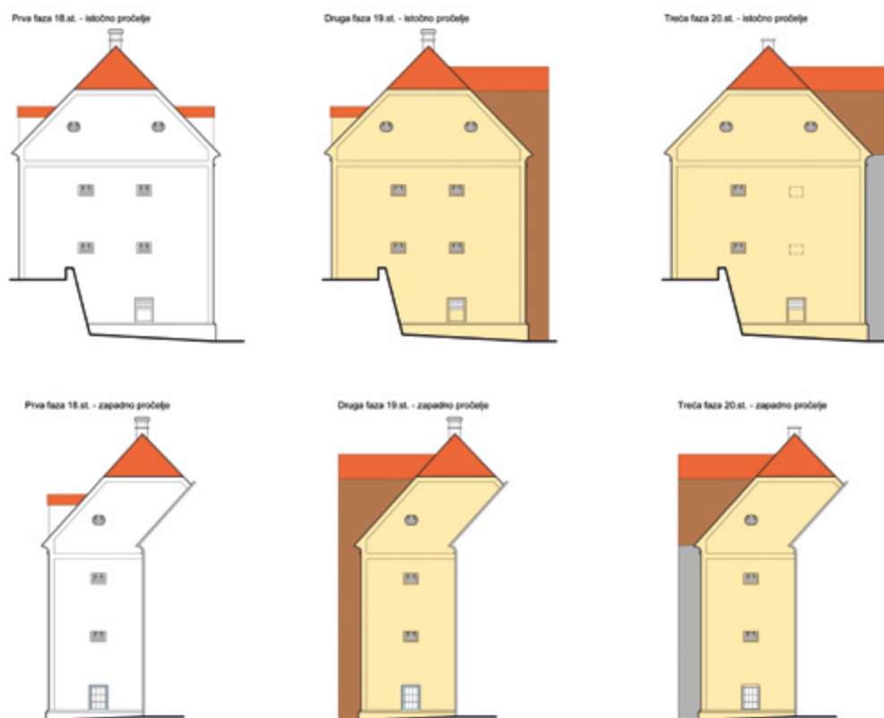
Sl. 20. Vojna pekara i skladište brašna, faze izgleda pročelja, istočno i zapadno pročelje (dokumentacija HRZ-a, podloge Urbos d.o.o., obradile I. Pauk Sili, V. Giener)
