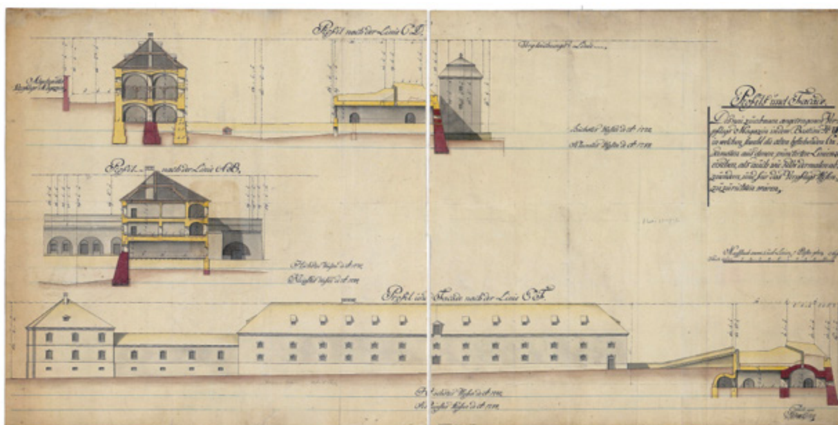
Sl. 4. Presjeci i pročelja za novoizgrađeni Opskrbni magazin u bastionu br. VIII, 1785. (Nacionalna i sveučilišna knjižnica u Zagrebu) Cross-section and façade for the newly built Supply Barracks in Bastion VIII, 1785 (National and University Library in Zagreb)
