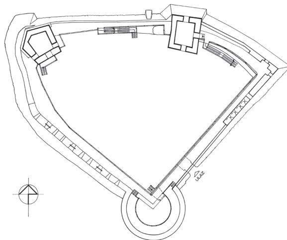
22. Kostajnica, Stari grad, prezentacija, tlocrt Kostajnica, Old Town, presentation, layout
