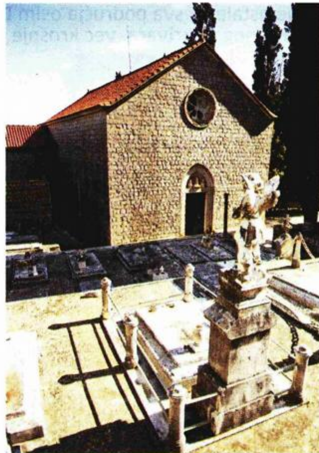
Crkva Gospe od Šunja potječe s početka 12. stoljeća
