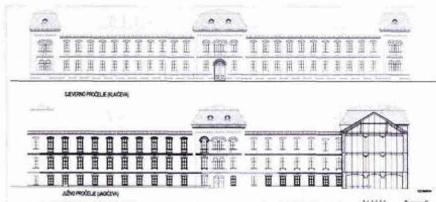
Crtež rekonstruiranoga sjevernog i južnog pročelja krila zgrade uz Klaičevu ulicu
