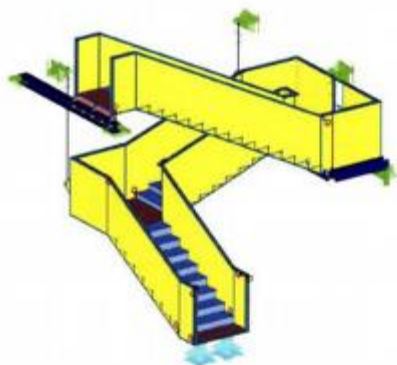
Prostorni FE model ovješeno stubište
