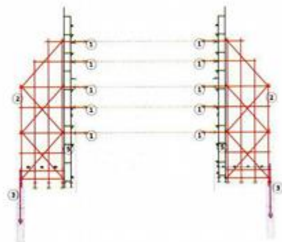
Vanjsko podupiranje postojećih zidova u fazi uklanjanja i građenja
