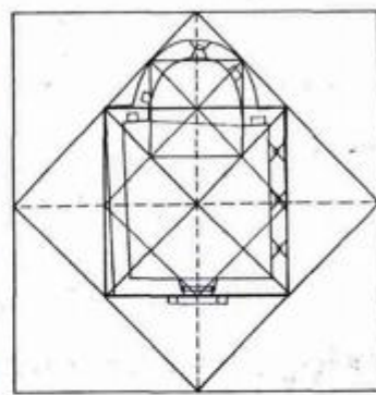
Tlocrt crkve određen je geometrijskom shemom kvadrangulacije
