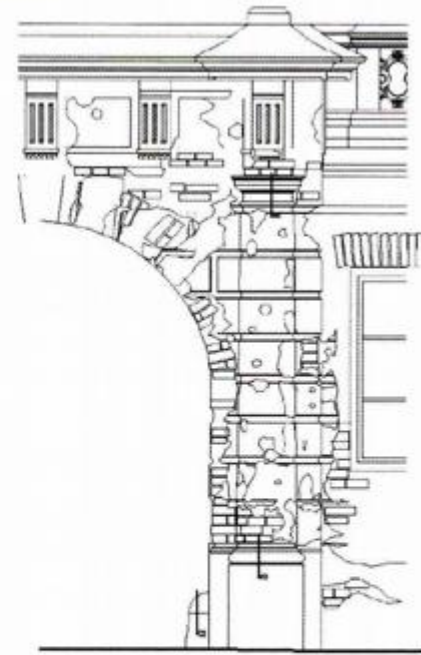
Crtež vrata s dekorativnim detaljima
