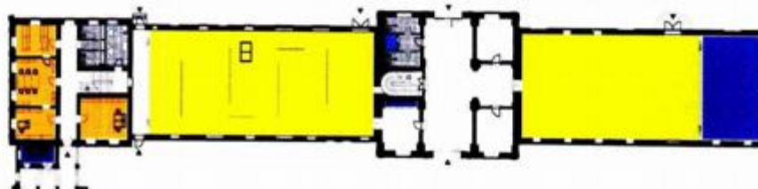
Tlocrt prizemlja Paviljona za goste
