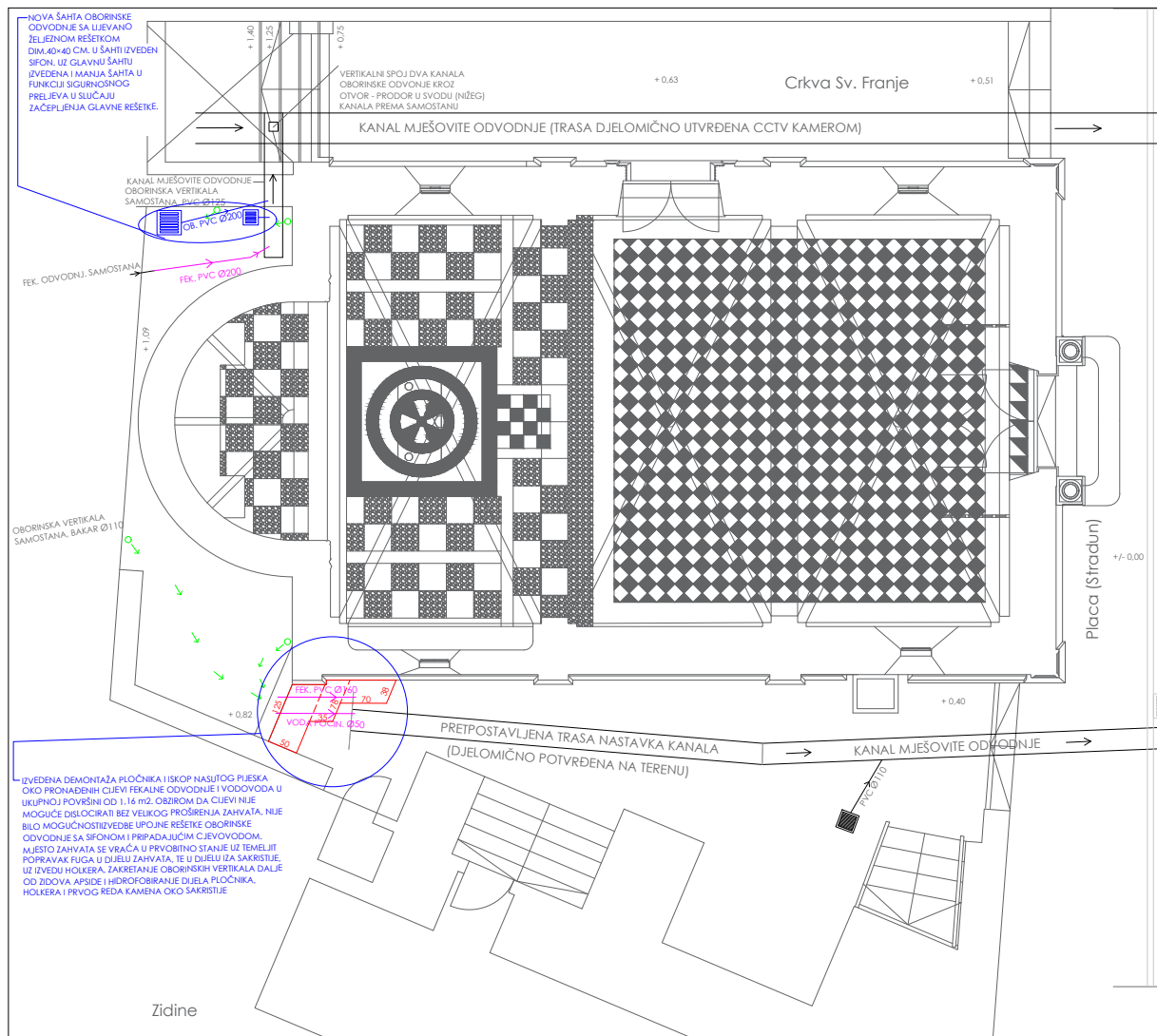
Dubrovnik, crkva Sv. Spasa, skica rješenja odvodnje oborinskih voda. Izrada: Dom izgradnja d.o.o., 2023. .
