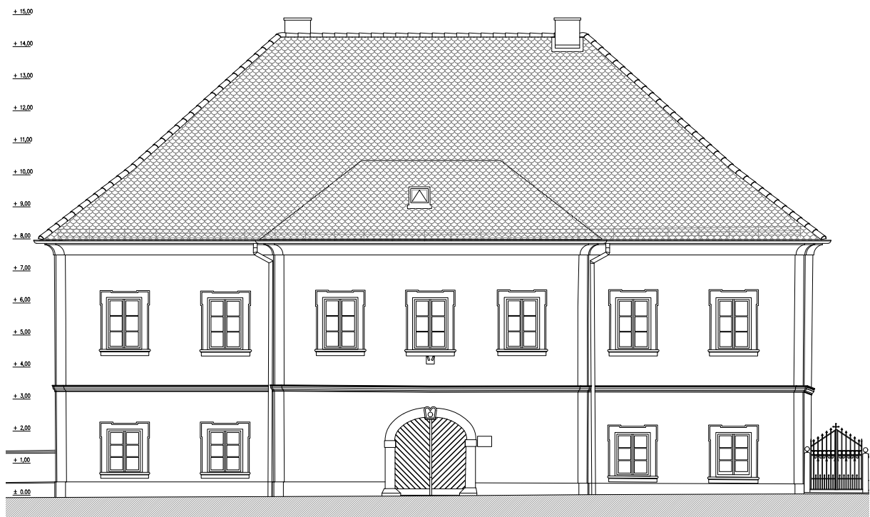
Sela, župni dvor crkve sv. Marije Magdalene. Projekt rekonstrukcije, adaptacije i opremanja prostora privremene čuvaonice, sjeverno pročelje. Izrada: A. Škevin Mikulandra, 2023.
