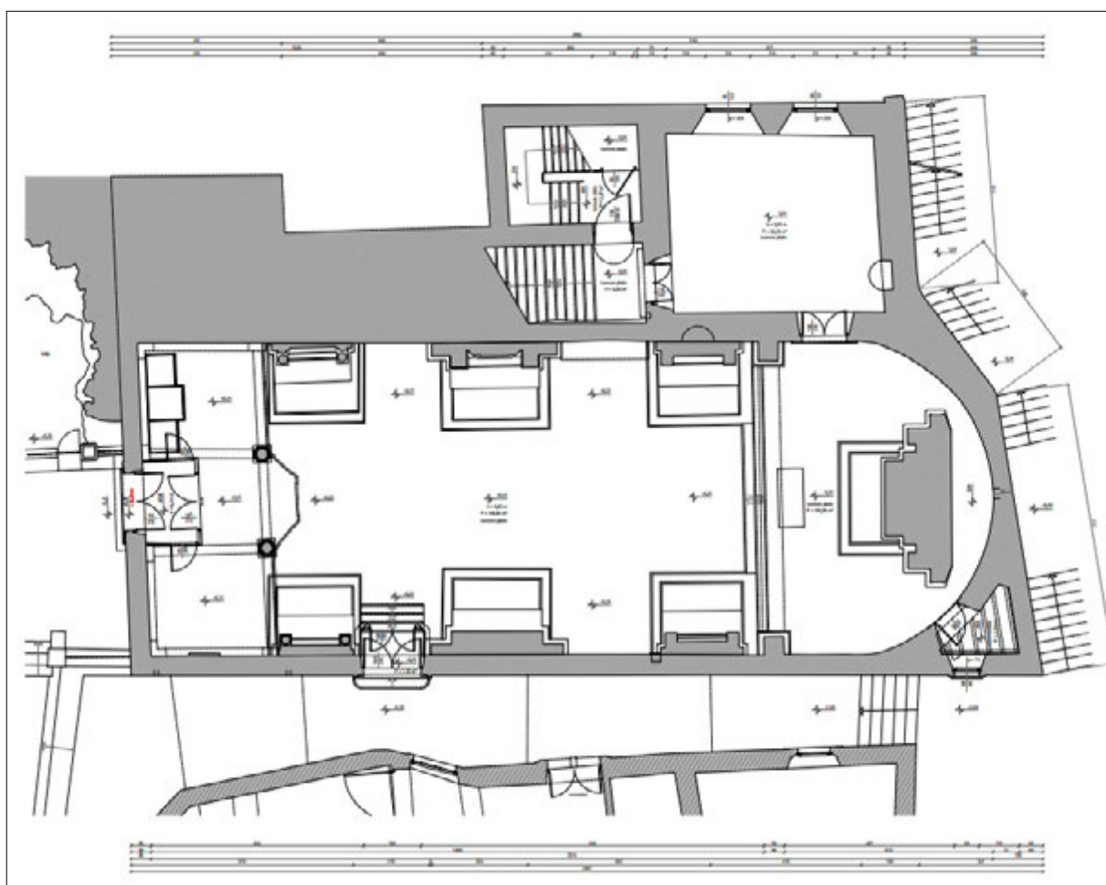
Šibenik, crkva sv. Lovre, tlocrt prve razine. Izrada: Skimi d.o.o., 2023.
