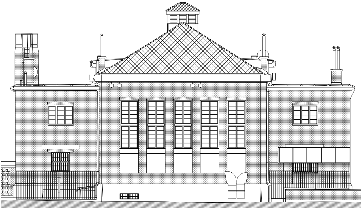
Zagreb, kompleks zgrada „Hrvatskoga sokola“ i „Kola“. Arhitektonska snimka postojećega stanja, južno pročelje. Izrada: SKIMI64 d.o.o., 2023.
