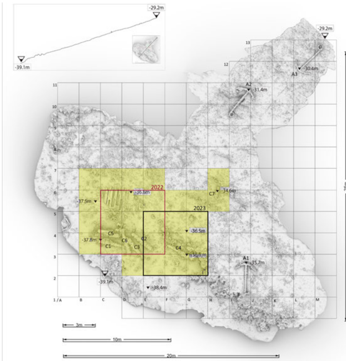
Otok Kornati, Bisage. Plan nalazišta i područje iskopa u 2022. i 2023. godini. Snimka: J. Macura i V. Zmaić, 2023.
