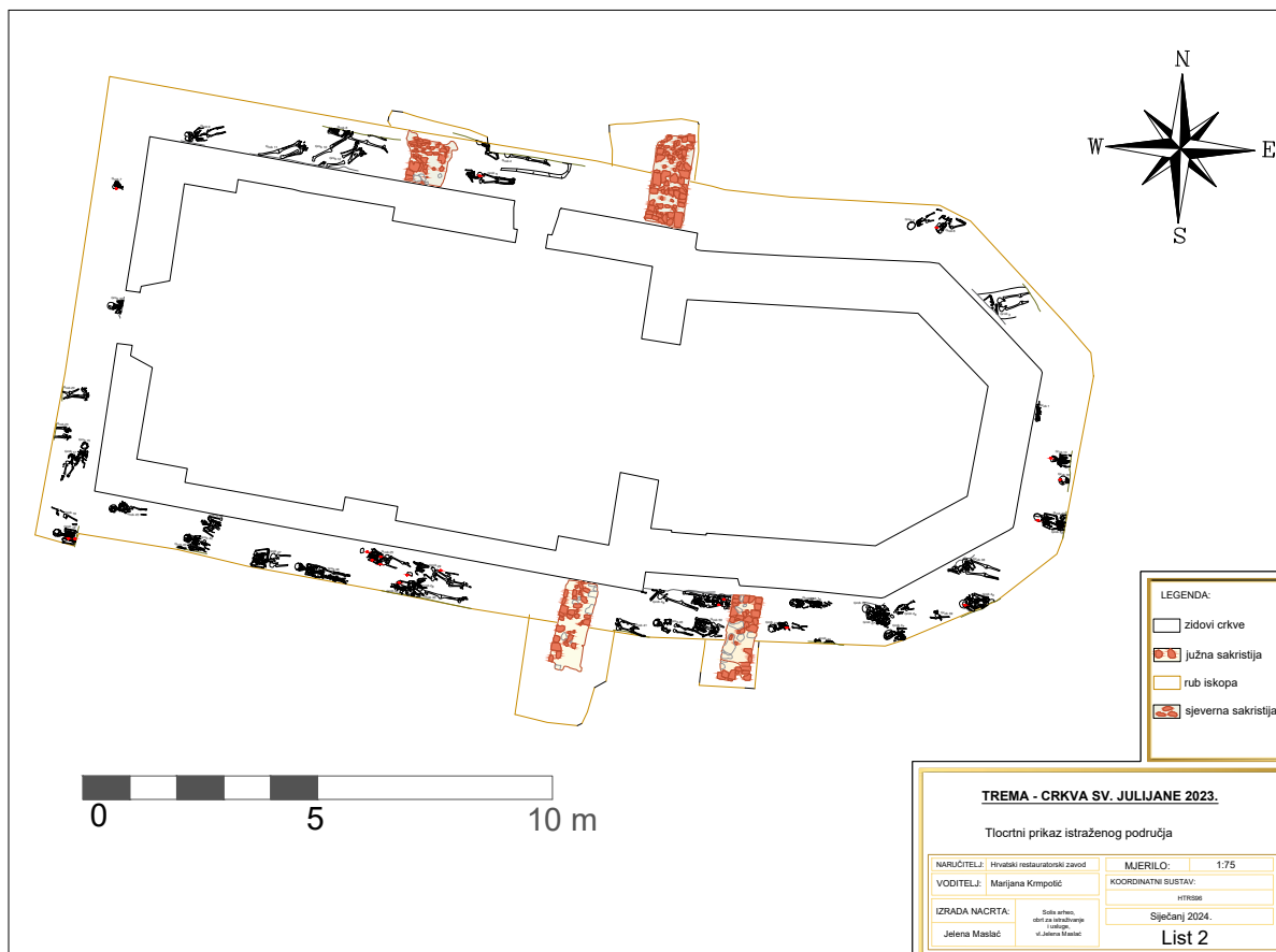
Trema, crkva sv. Julijane, tlocrtni prikaz istraženoga područja. Izrada: J. Maslač, 2023.
