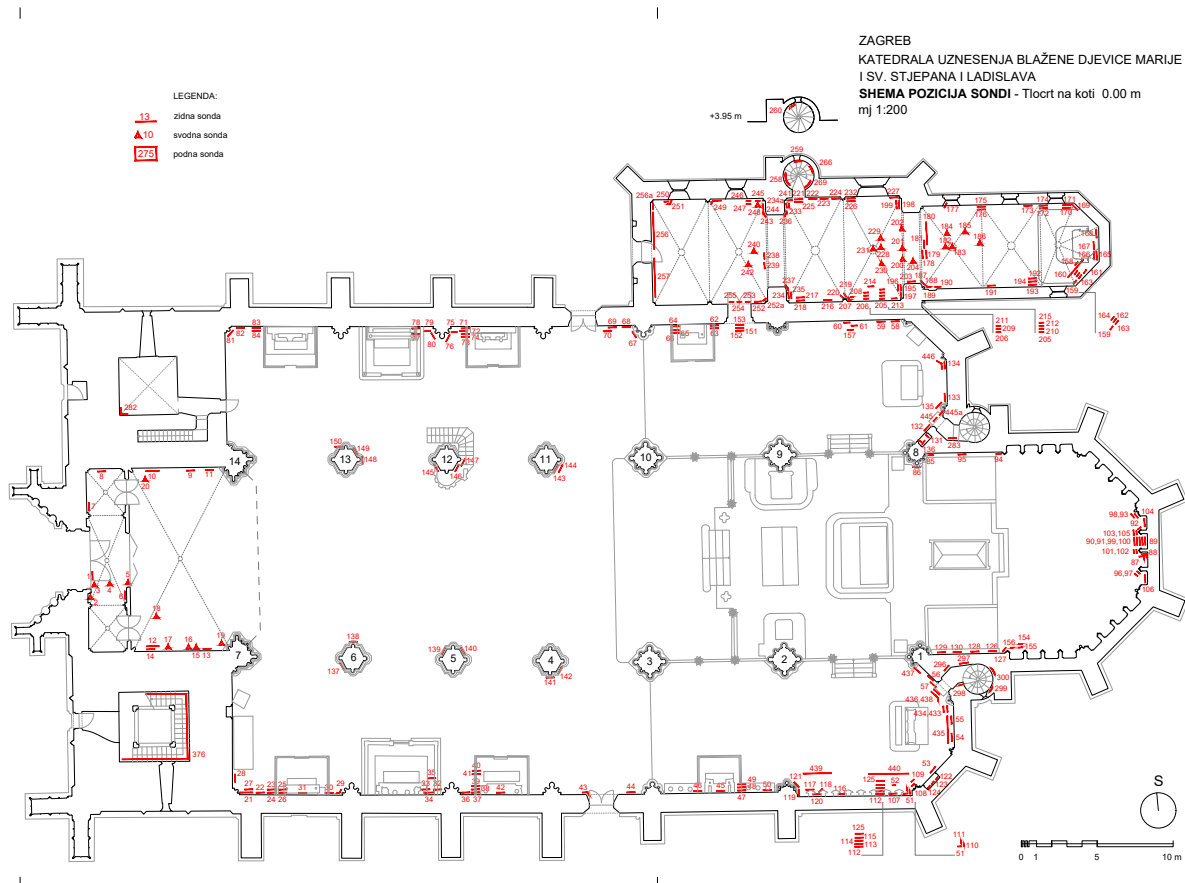
Zagreb, Kaptol, katedrala Uznesenja BDM i sv. Stjepana i Ladislava. Tlocrt prizemlja, pozicije sonde. Izrada: K. Majer Jurišić, K. Krulić, M. Deak, T. Prpić, 2023.
