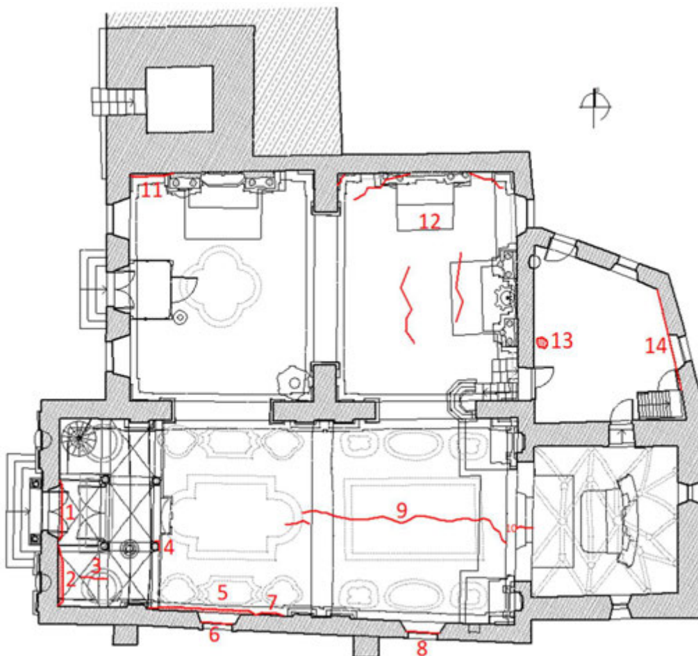
Lovran, crkva sv. Jurja, tlocrt prizemlja, nacrt oštećenja konstrukcije. Izrada: Intrados projekt d.o.o., 2023.
